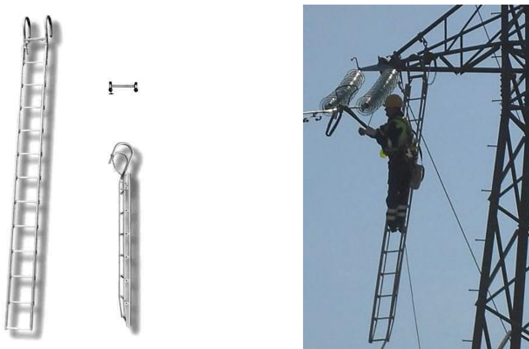
122.-123. Függesztő létra
